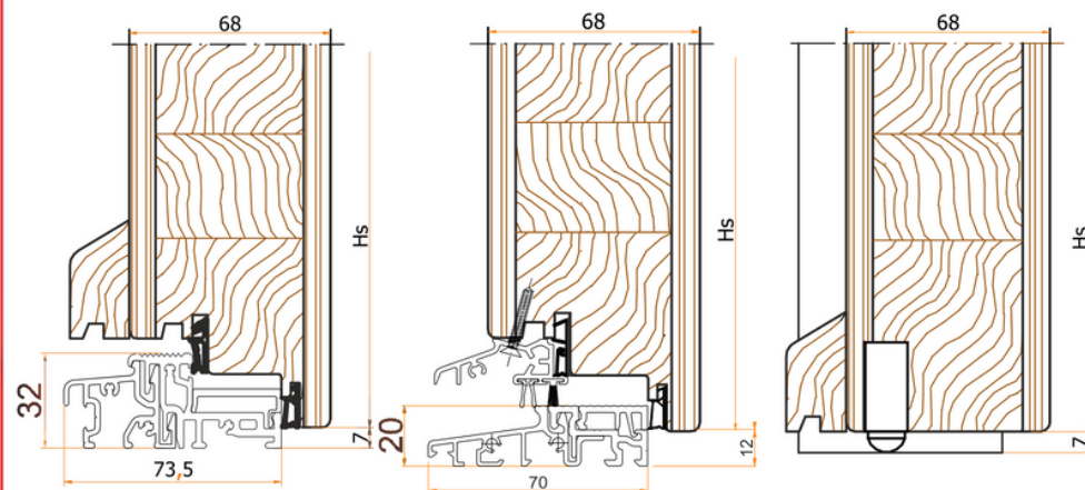
Próg aluminiowy GUTMANN 74/32 TI
