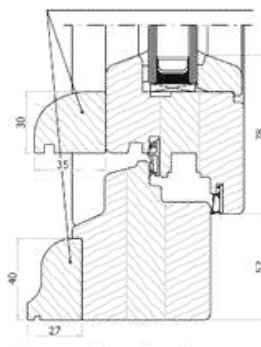
okapnik drewniany Belgijski
