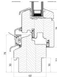
okapnik aluminiowy
