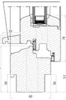
okapnik drewniany skrzydła
